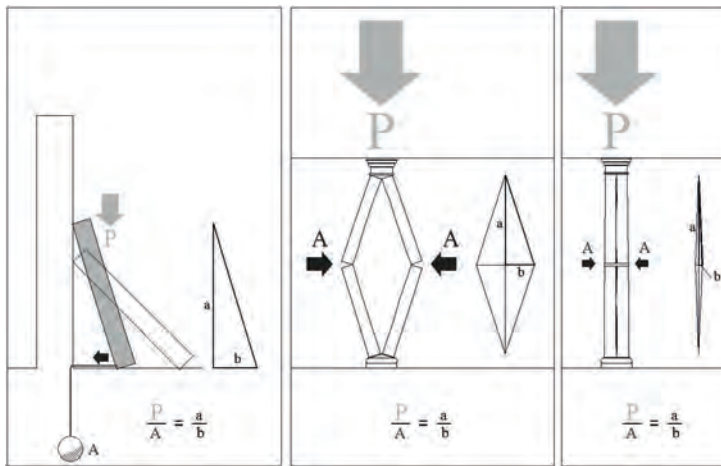
Abb. 2.103: Evangelista Torricelli, Reparatur gerissener Säulensäfte (Graphik: H. Schlimme).
