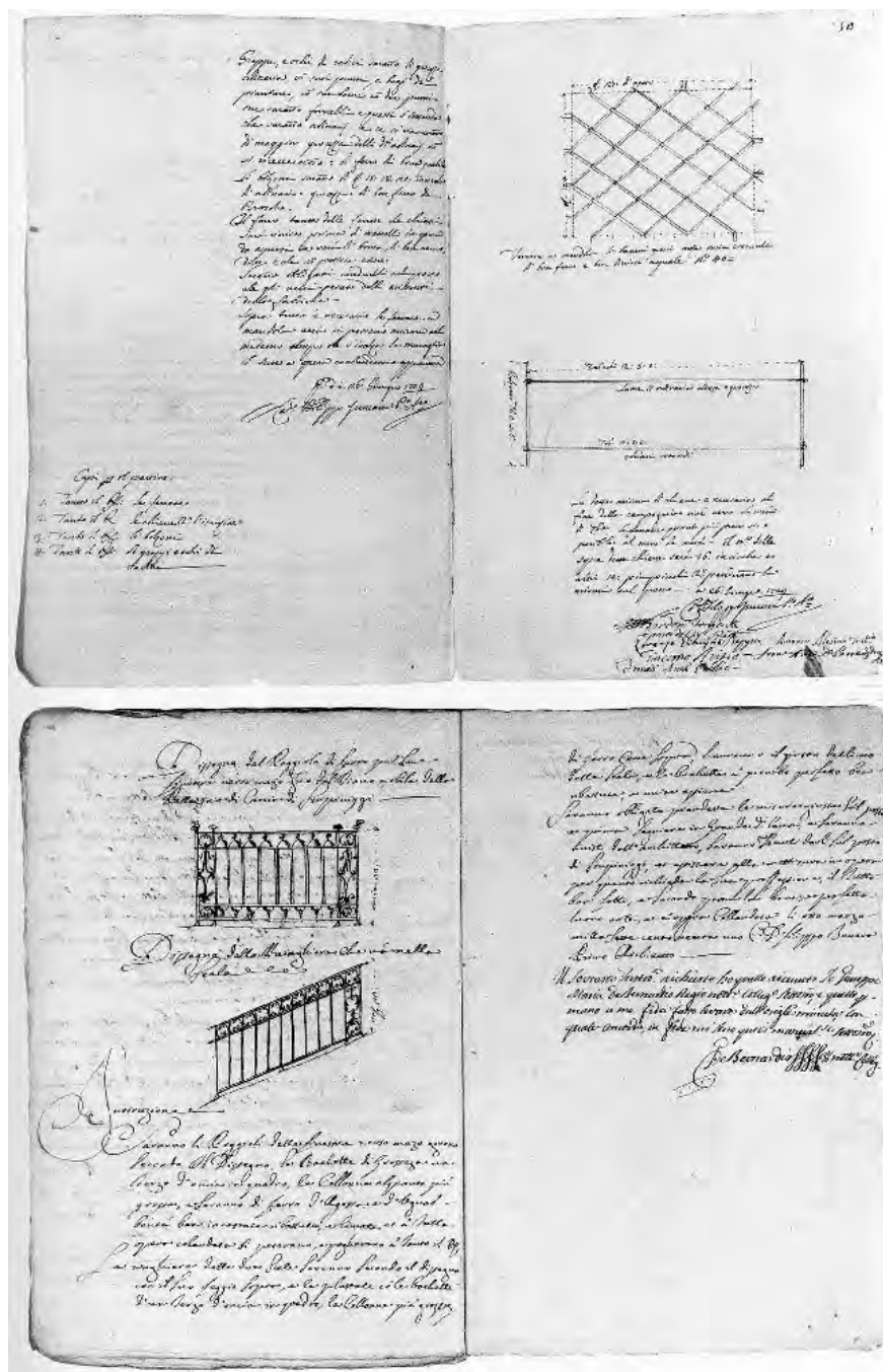
Abb. 2.40: Filippo Juvarra, Erläuterungen und Zeichnungen für Schmiedeeisenarbeiten für das Schloss in Stupinigi, 1729, 1731 (Archivio Storico della Fondazione Ordine Mauriziano, Turin, Minutario De Bernardis, 1727 a 1731, n. 9, c. 30 [oben] und Stupinigi, Mazzo 14, c. 461 [unten]).
