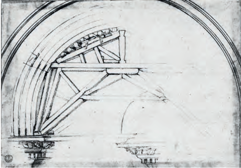
Abb. 2.78: St. Peter, Rom, Lehrgerüst für die kuppeltragenden Bögen, Datierung wird nachgetragen, Uff. A 226 (Gabinetto Disegni e Stampe degli Uffizi, ; mit Erlaubnis des Ministero dei Beni e delle Attività Culturali e del Turismo; Reproduktion nicht gestattet).
