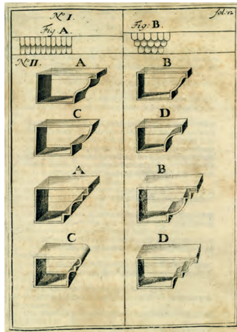
Abb. 5.3: Formen der Dachziegel und der Deckungen. Figur A zeigt die sogenannte einfache, Figur B die doppelte Deckung des Daches. Die anschließend dargestellten Gesime sollten dem Bauherrn veranschaulichen, welche standesgemäßen Formen angemessen seien (Böckler 1678, zwischen S. 12 und S. 13).
