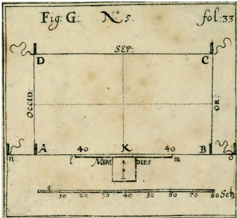
Abb. 5.6: Darstellung eines aufgeschnürten Bauplatzes des Wohnhauses (Böckler 1678, zwischen S. 32 und S. 33).
