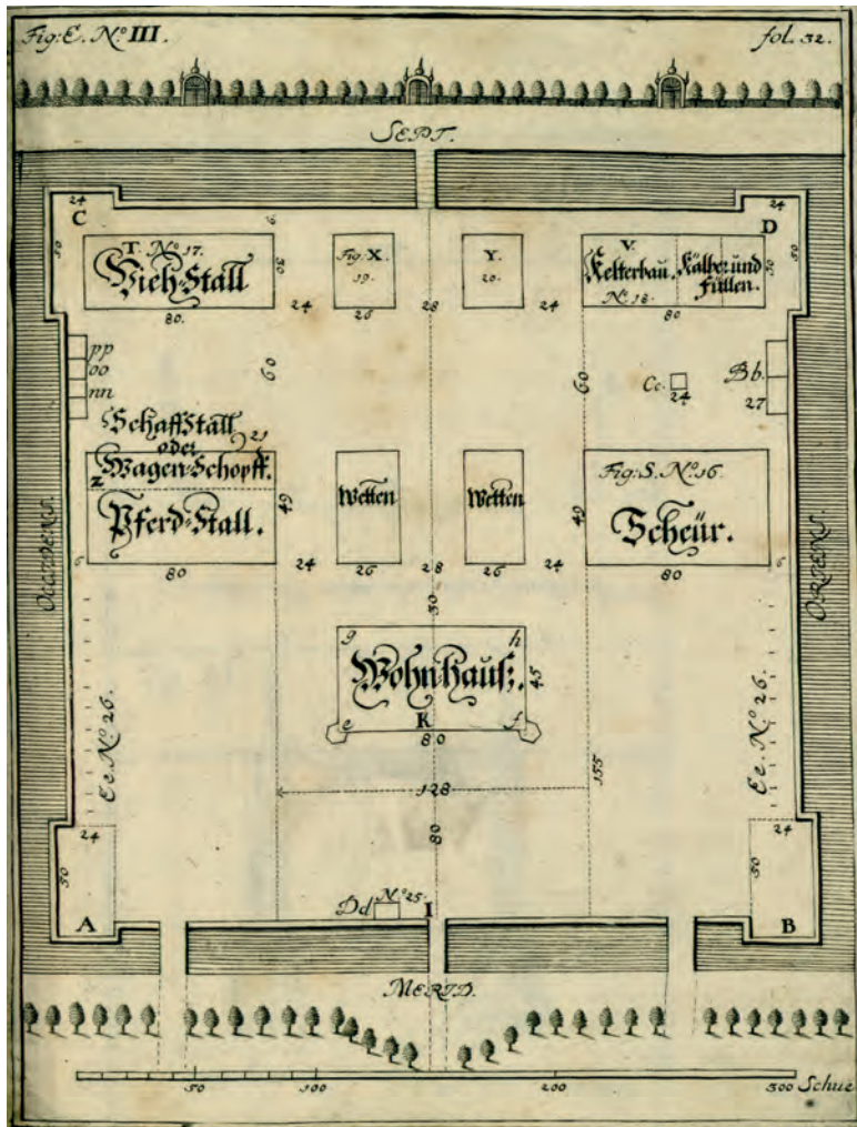
Abb. 5.5: Vermaßter und genordeter Detailplan der Funktionsgebäude eines adligen Meyerhofes (Böckler 1678, zwischen S. 32 und S. 33).
