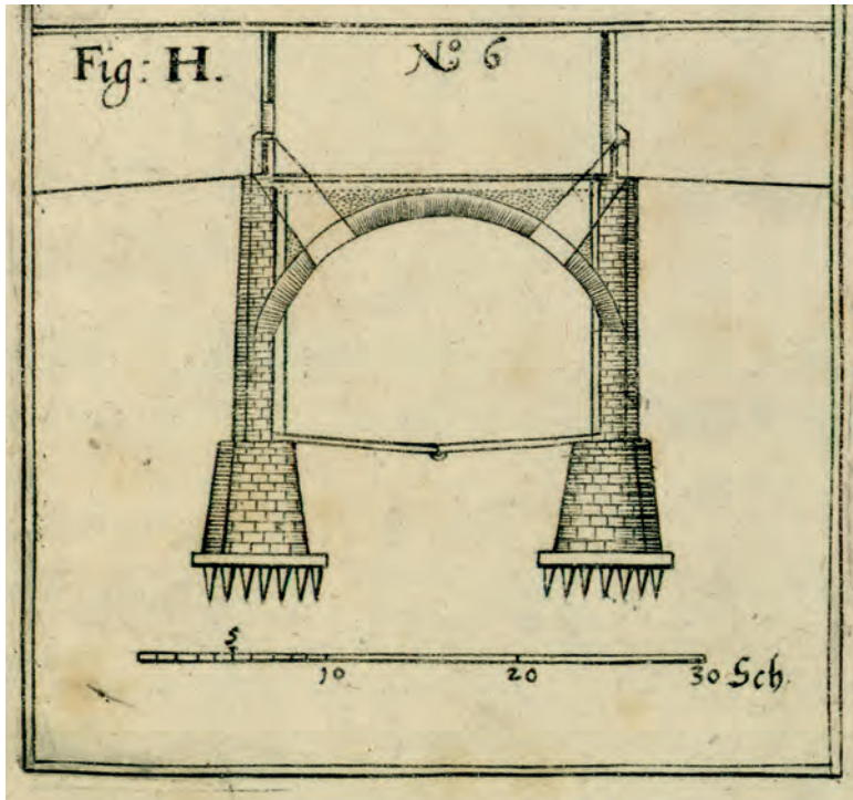
Abb. 5.7: Schnitt durch ein Fundament (Böckler 1678, zwischen S. 32 und S. 33).
