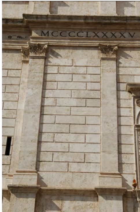
Abb. 2.66: Palazzo della Cancelleria, Rom, ab 1486, Fassadendetail (Foto: H. Schlimme).
