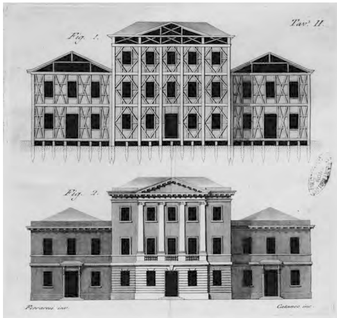
Abb. 2.17: Vincenzo Ferraresi, Entwurf eines antiseismischen Hauses, Fassadenaufriss und Querschnitt, aus: Vivenzio 1783 (Biblioteca Nazionale Centrale di Roma, mit Erlaubnis des Ministero dei Beni e delle Attività Culturali e del Turismo; Reproduktion nicht gestattet).
