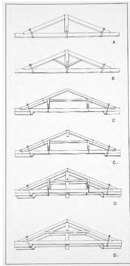
Abb. 2.89: Simona Valeriani, Die Grundtypen der in Mittelitalien vorkommenden Dachwerke: A einfaches Hängewerk, B Hängewerk mit Spriegen, C einfache palladiana mit seitlichen Hängesäulen, C1 einfache palladiana mit mittlerer und seitlichen Hängesäulen, D doppelte palladiana mit seitlichen Hängesäulen, D1 doppelte palladiana nur mit mittlerer Hängesäule (Quelle für Abbildung und Bildunterschrift: Valeriani 2006, 31, mit freundlicher Erlaubnis).
